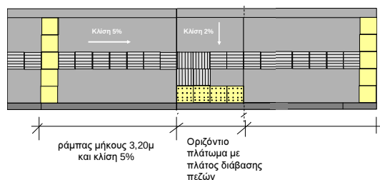
Ράμπα σε πεζοδρόμιο ύψους 17 εκ.
