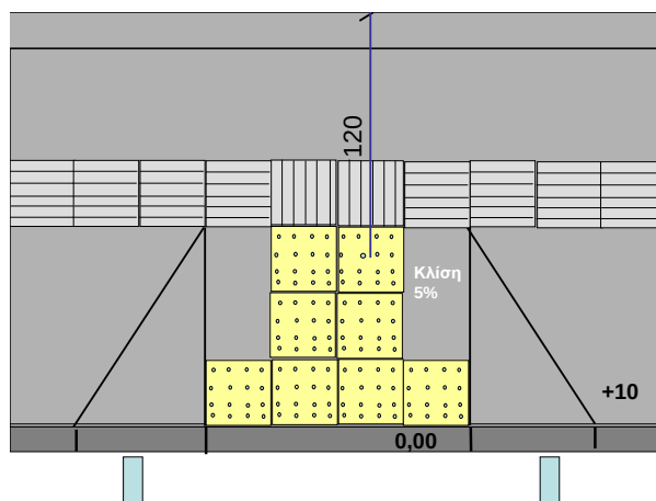
Ράμπα κάθετη προς τη διεύθυνση του πεζοδρομίου, με οριζόντιο πλάτωμα στο πάνω μέρος
