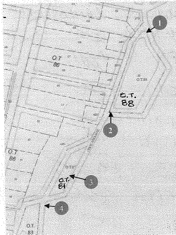
Εγκεκριμένο Ρυμοτομικό Σχέδιο
